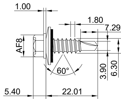
TSFHR6.3-22-2
